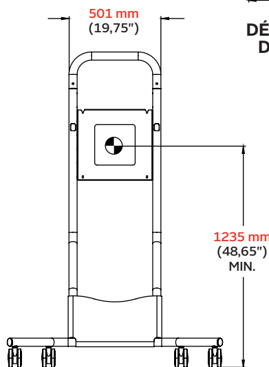
VUE AVANT
