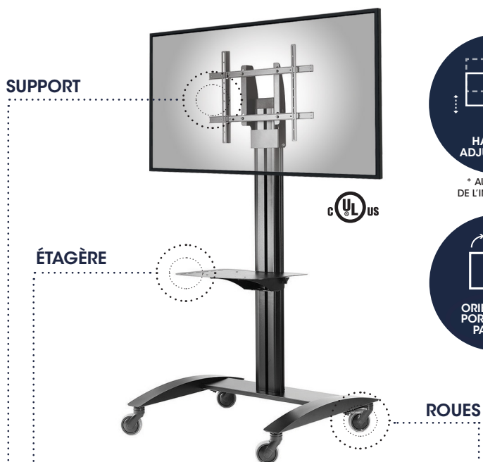
Chariot pour écran plat de 32" à 75" SR560M
