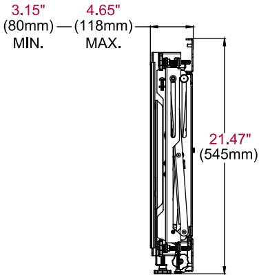
VUE LATÉRALE RÉDUITE
